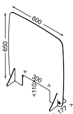
Malý model se stojanem
