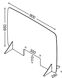
Velký model se stojanem
