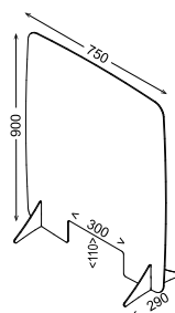
Zvýšený model se stojanem
